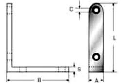
EY08076E S/S AISI 304 STAMPED CORNER BRACKET 70X70 (R3S510)
